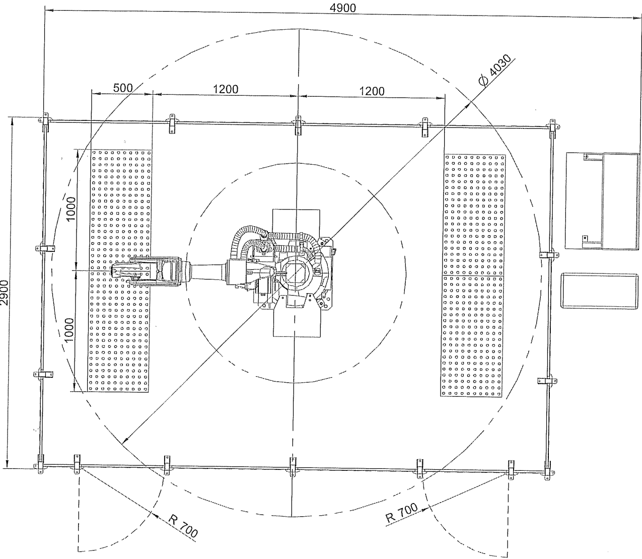
schema a rozměry pracoviště (místo dveří vstup jištěn světelnou závorou)
